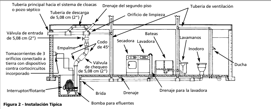
Figura 2 - Instalación Típica
